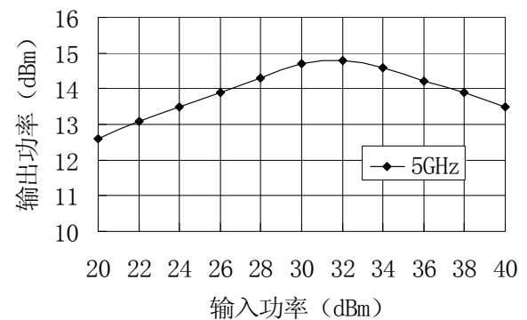
限幅电平
