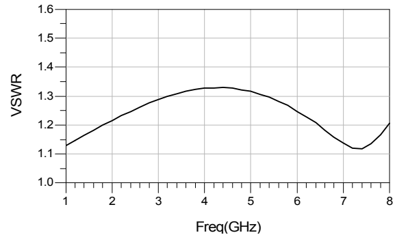
输入/输出驻波 vs. 频率
