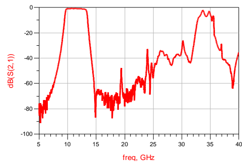
远端抑制 VS 频率(T A =25°C)
