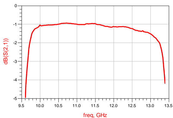
通带损耗 VS 频率(T A =25°C)
