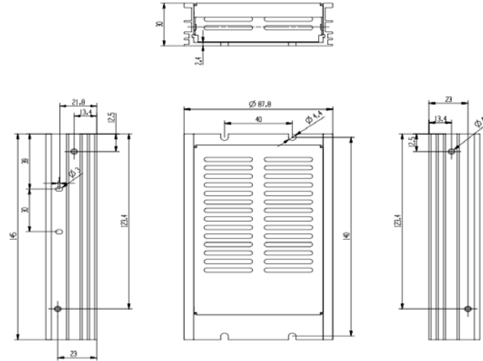
图 1-1 安装及尺寸图
