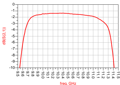
通带损耗 VS 频率(T A =25°C)
