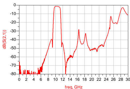
远端抑制 VS 频率(T A =25°C)
